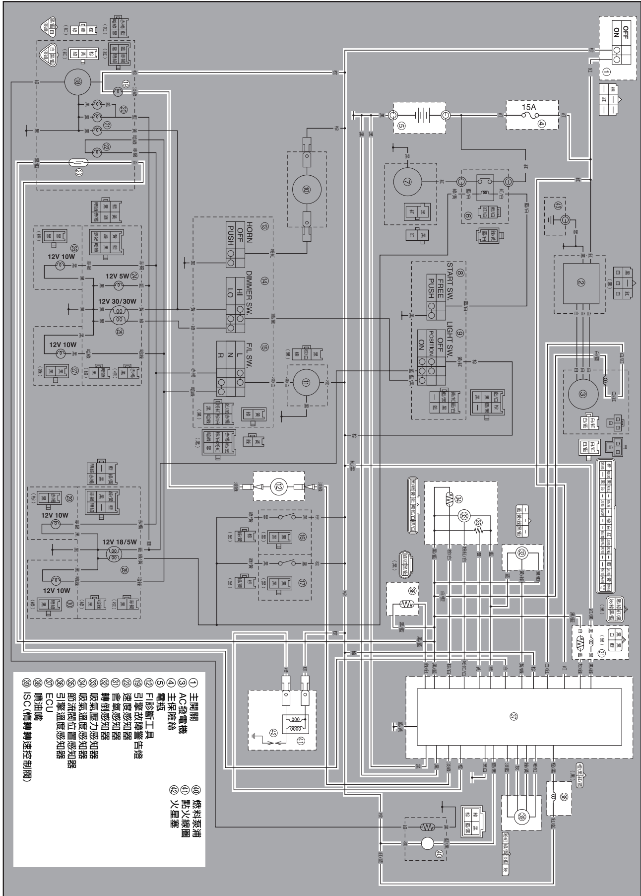
線路圖(37C2)
