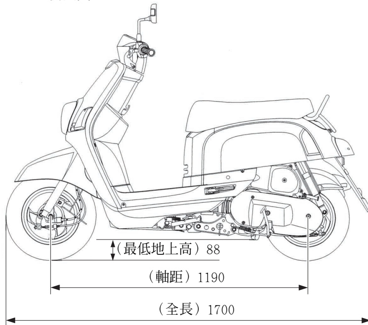
側面圖
