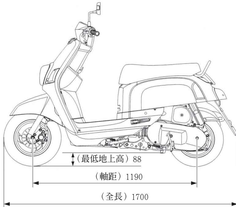
側面圖
