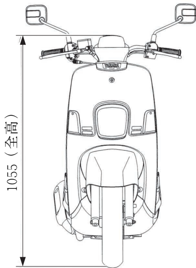
前面圖
