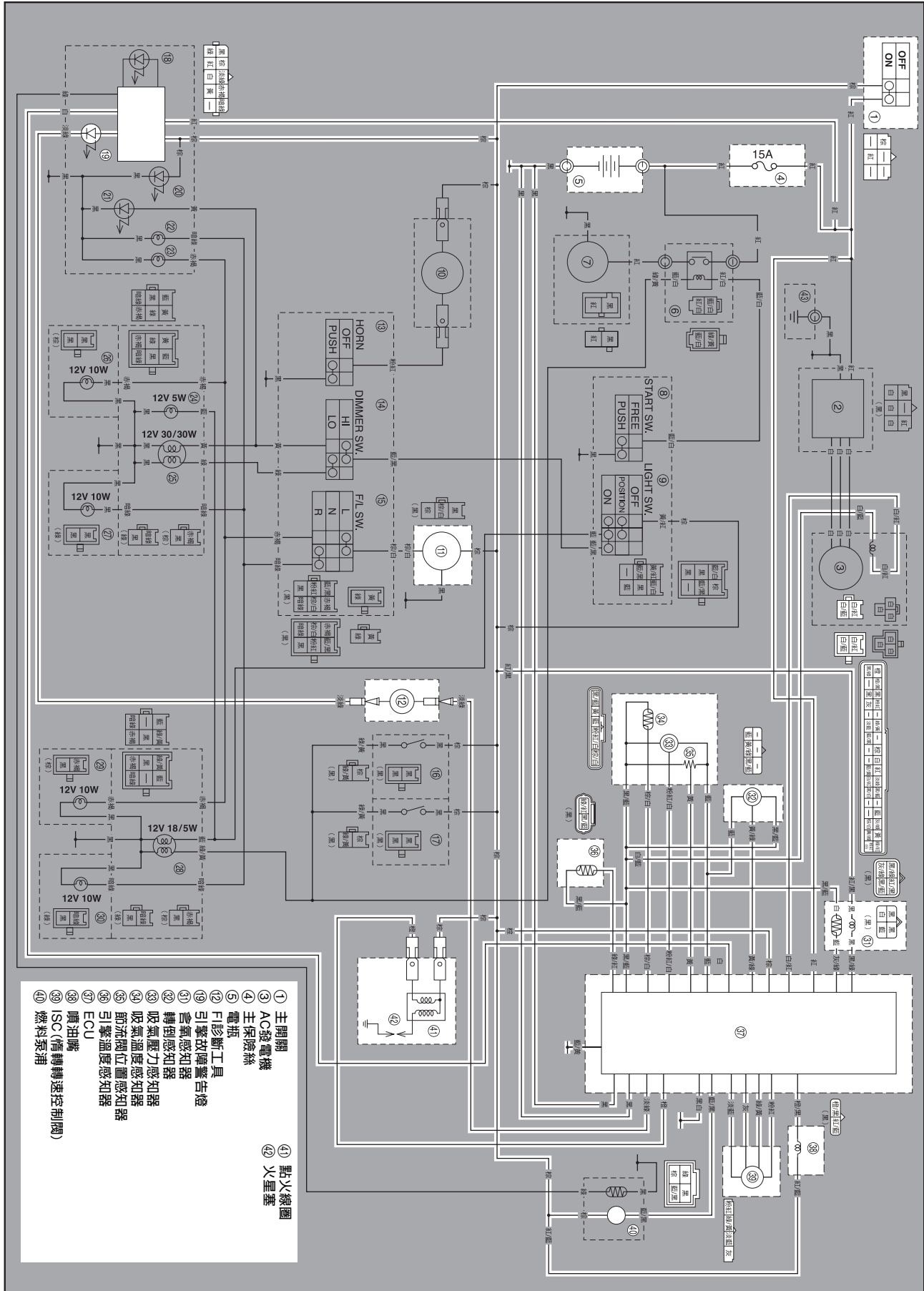
線路圖(37C1)
